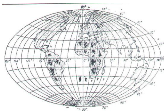
Grintenova projekcija
