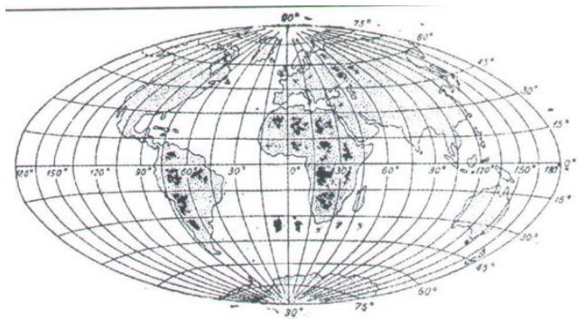
Ajtovljeva projekcija
