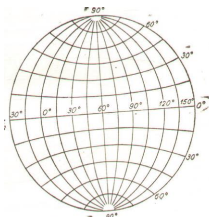
Loptasta projekcija
