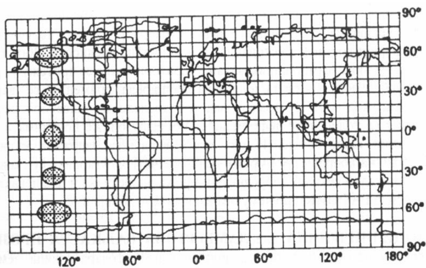
Kvadratna projekcija
