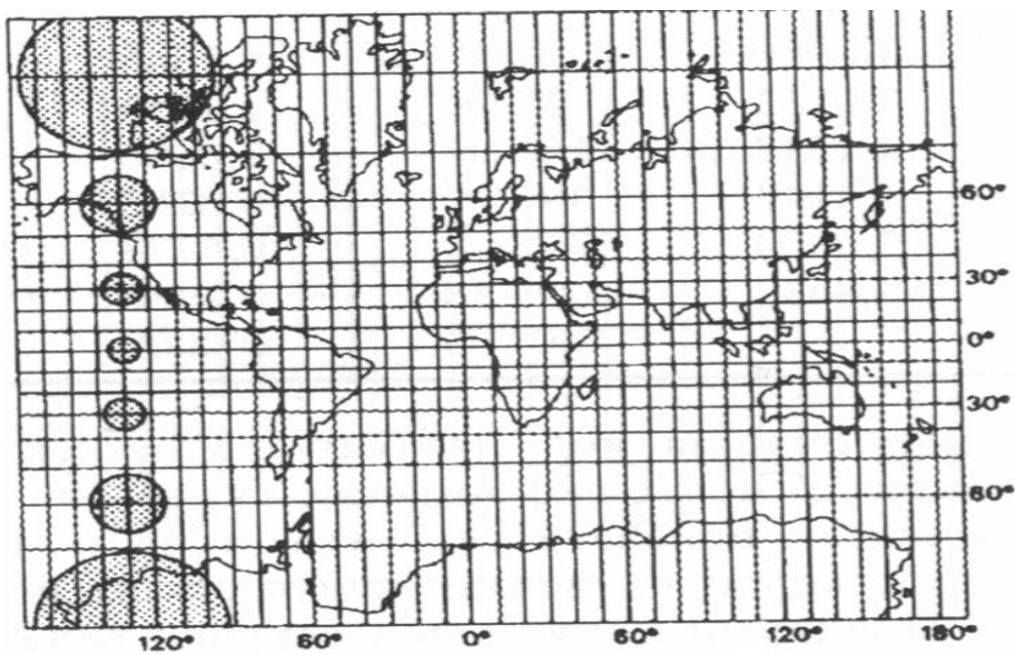
Merkatorova projekcija
