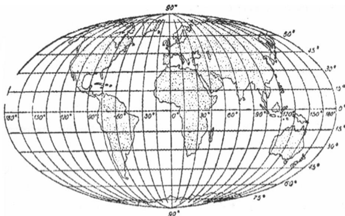
Molvajdeova projekcija
