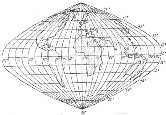
Sansonova projekcija
