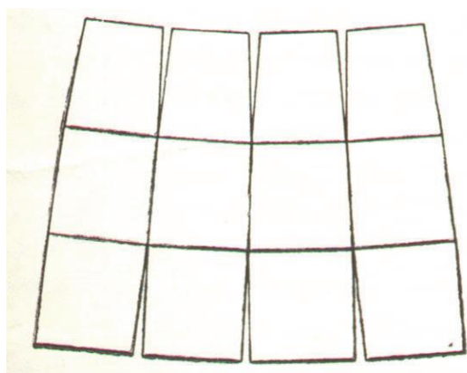
Loptasta projekcija
